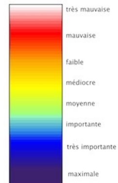
Qualité du ciel et de l'environnement nocturnes en France métropolitaine
